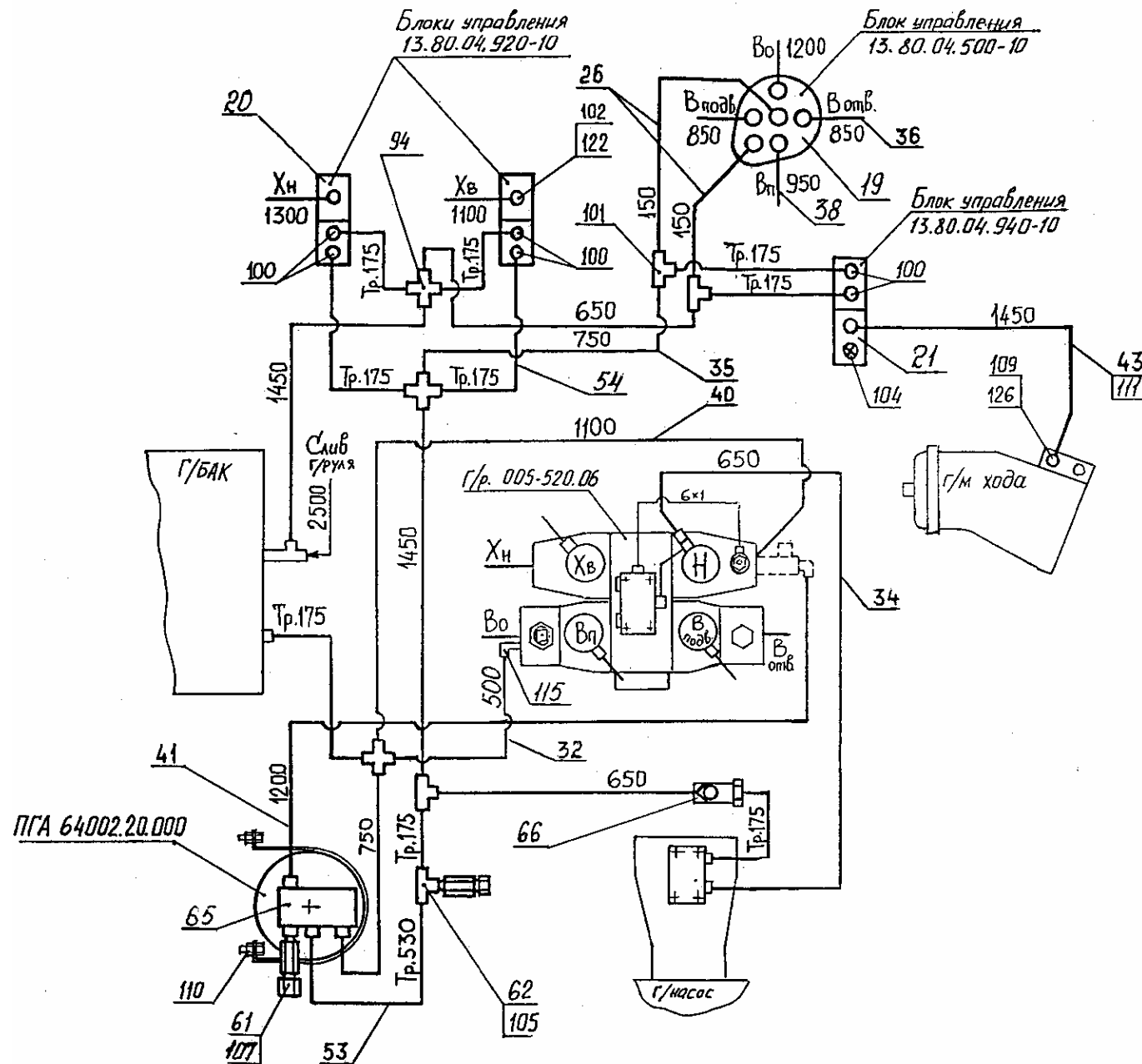
Рис. 34.1 Гидроуправление Fig. 34.1 Hydraulic Control System
