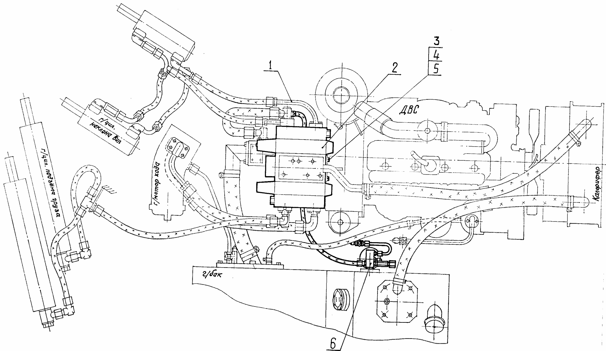
Рис. 19 Гидрооборудование Fig. 19 Hydraulic Equipment
