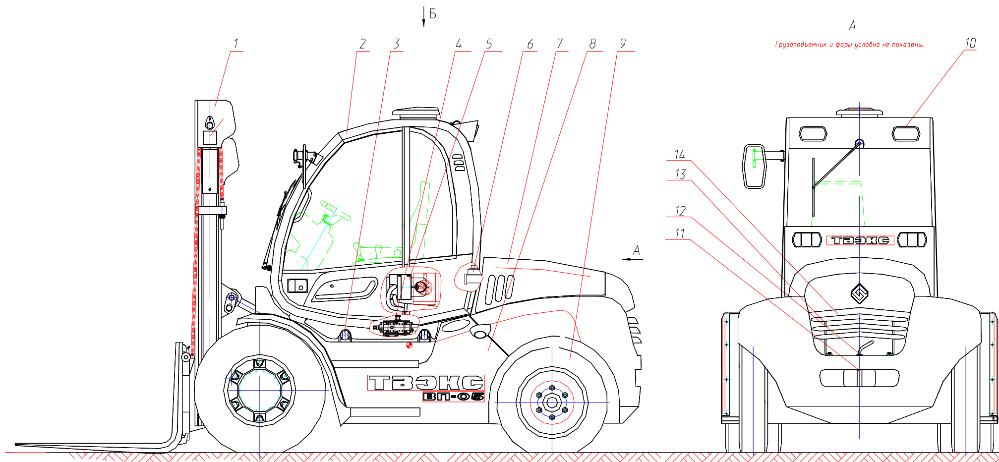
Рис. 1.1 Гидравлический вилочный погрузчик Fig. 1.1 Hydraulic Fork Loader
